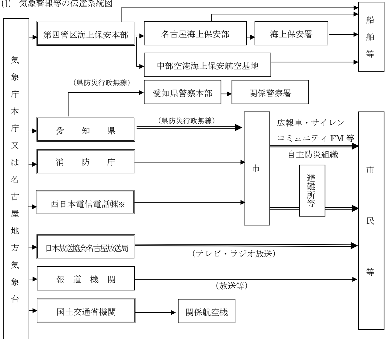
(1) 気象警報等の伝達系統図
