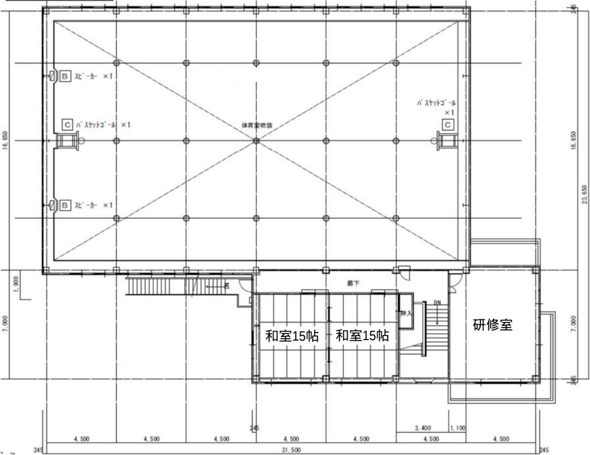
2階平面図
