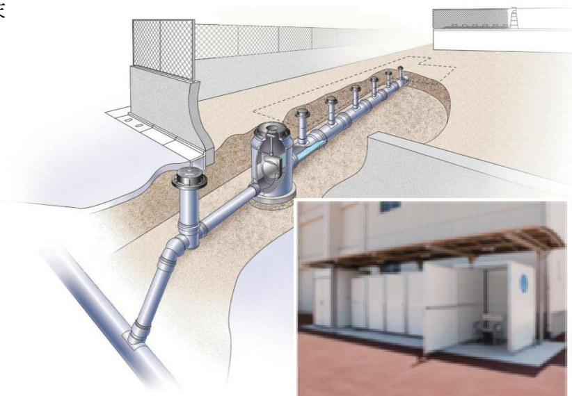
（参考例）駐輪場を利用したマンホールトイレ
