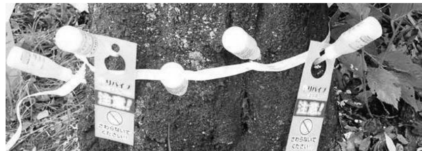
（写真31）樹幹注入の穴のあけ方 一定間隔にあけるところを決め、その上下にばらつかせてあける
