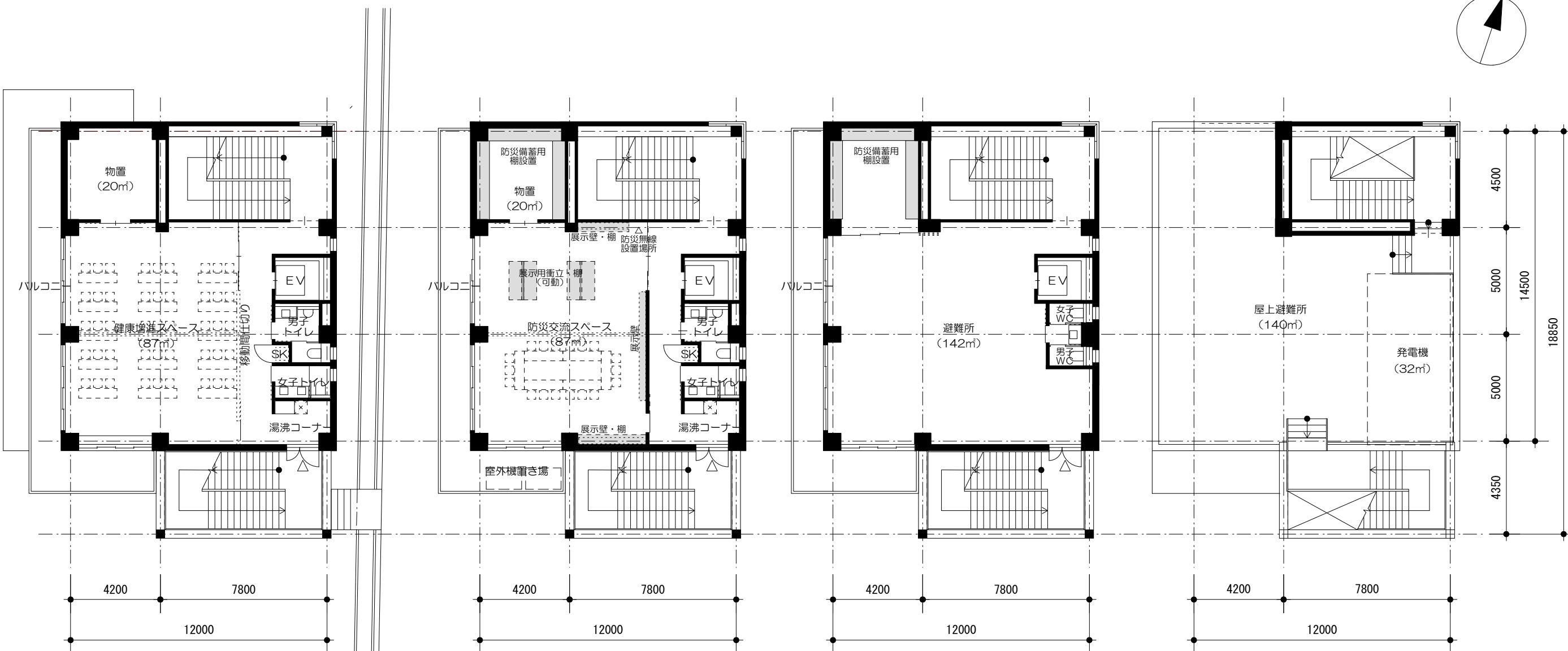
2階平面図
